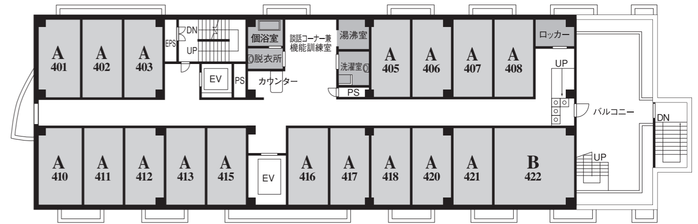
4階平面図
